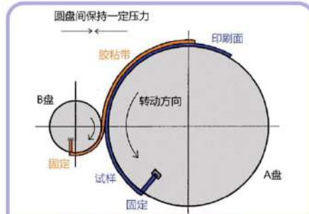
Gx-B2型圆盘剥离试验机 Gx-B2 Disk Stripping Tester
